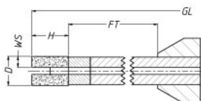
Werkzeugtyp Pos. 1
