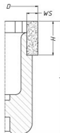
Werkzeugtyp Pos. 9, 10
