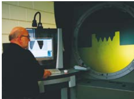
Die Endkontrolle stellt sicher, dass das Profil eines Grundkörpers allen Zeichnungsanforderungen entspricht.
