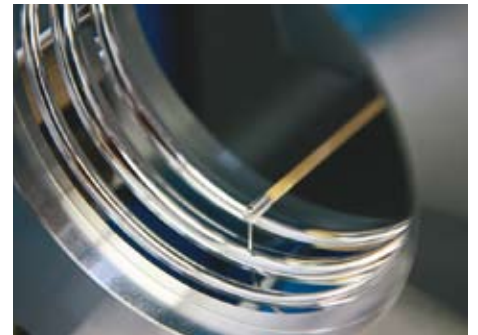
Mikrometergenaue Vermessung des Profils einer Negativform für Diamant-Abrichtrollen.
