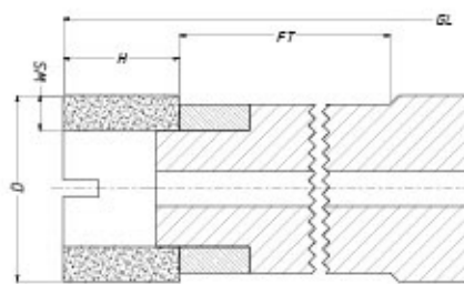
Werkzeugtyp Pos. 2-4
