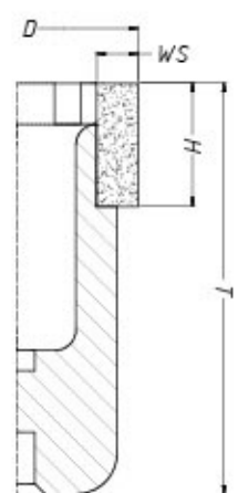
Werkzeugtyp Pos. 9, 10
