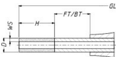
Werkzeugtyp Pos. 1, 2, 5, 6
