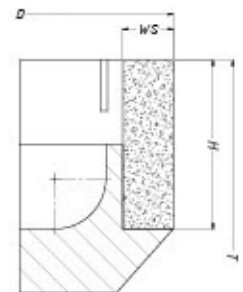
Werkzeugtyp Pos. 5-7
